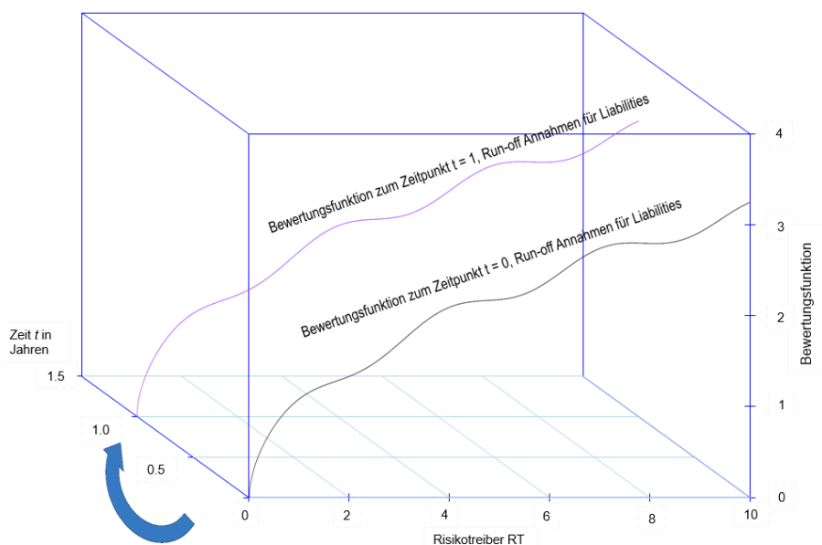
Abbildung 1 Approximation der Bewertungsfunktion zum Zeitpunkt bei t = 1 durch die zum Zeitpunkt t = 0
